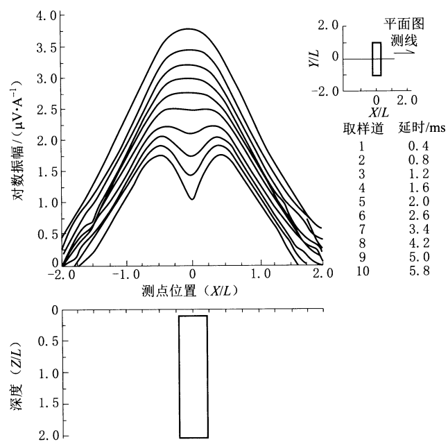
图 F.5 厚板模型的 TEM 曲线
