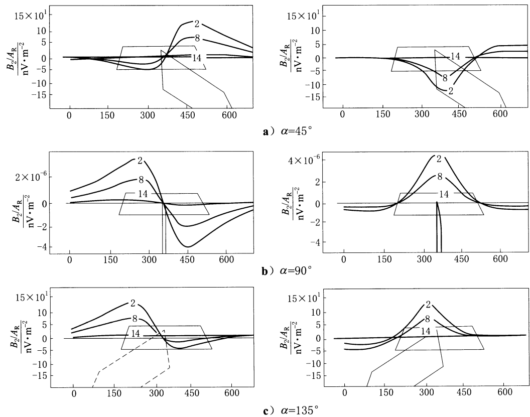
图 F.12 定源回线内、外不同倾角的导电薄板异常剖面曲线图
