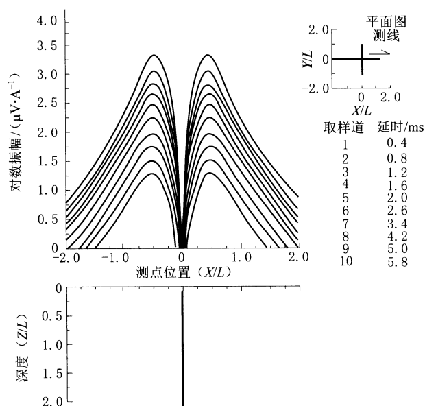
图 F.1 直立薄板模型的 TEM 曲线( \delta=90^\circ )
