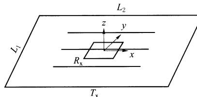
图 5 定源回线内工作装置示意图
