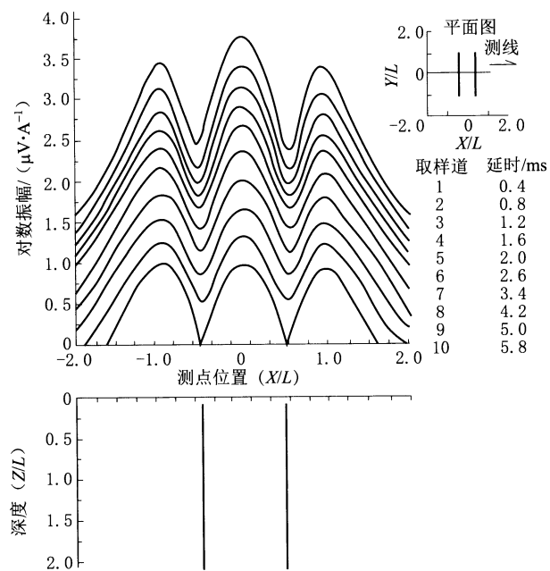
图 F.6 复合薄板模型的 TEM 曲线
