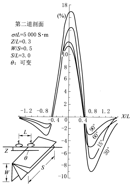
图 F.9 倾斜薄板 TEM 响应曲线
