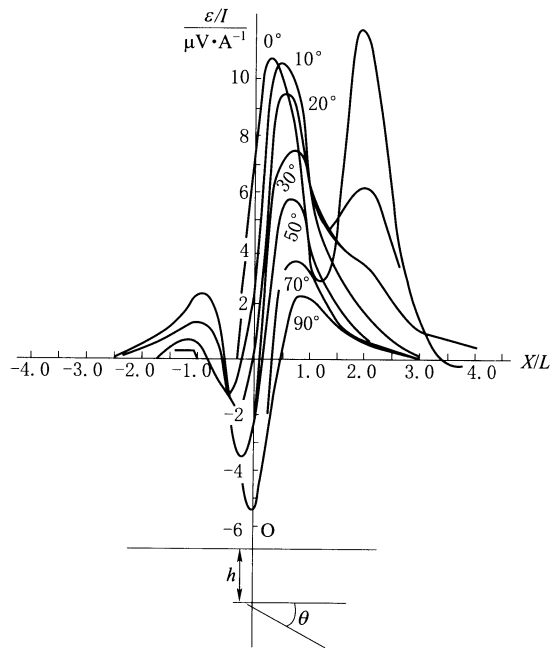
图 F.10 倾斜薄板的 TEM 响应曲线
