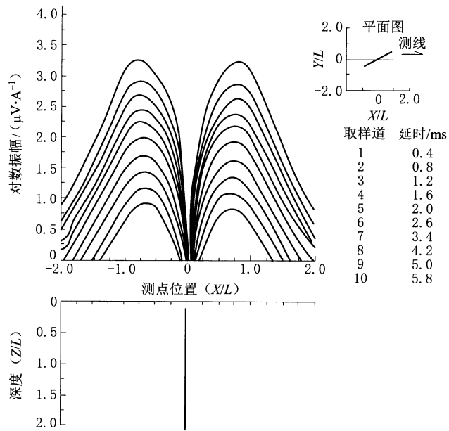
图 F.4 直立薄板模型的 TEM 曲线 ( \delta=90^\circ, \alpha=30^\circ )
