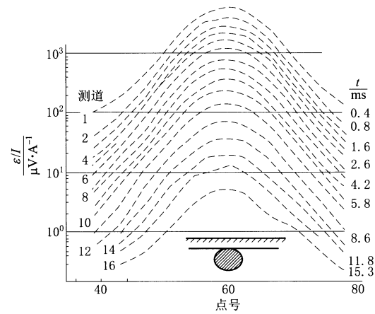
图 F.11 重叠回线水平圆柱体异常剖面曲线图
