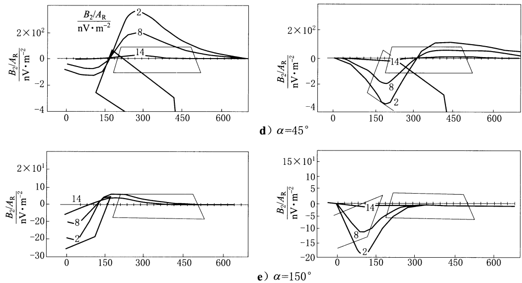
图 F.12 定源回线内、外不同倾角的导电薄板异常剖面曲线图(续)
