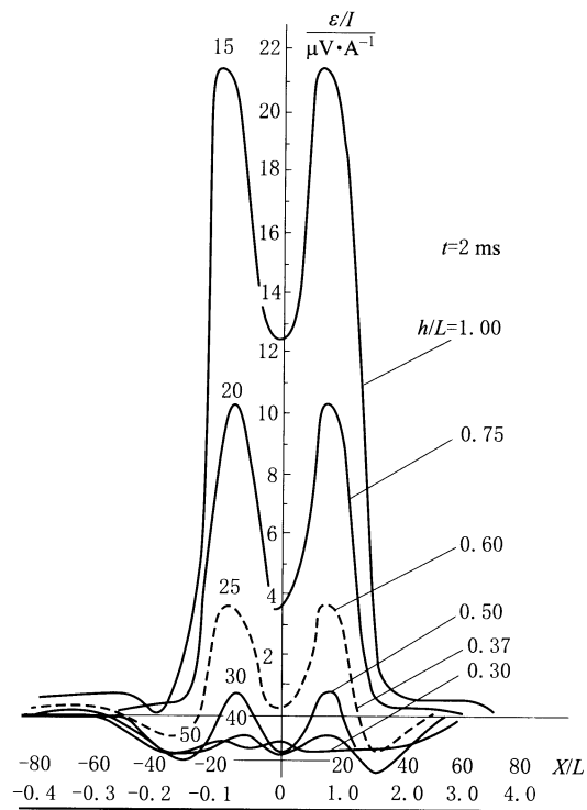
图 F.8 水平薄板的 TEM 响应曲线
