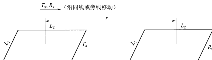
图 3 偶极装置示意图
