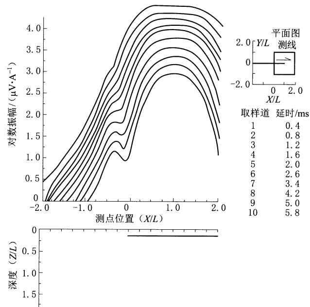
图 F.3 水平薄板模型的 TEM 曲线 ( \delta=0^\circ )
