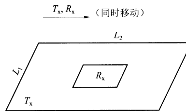
图 2 中心回线装置示意图
