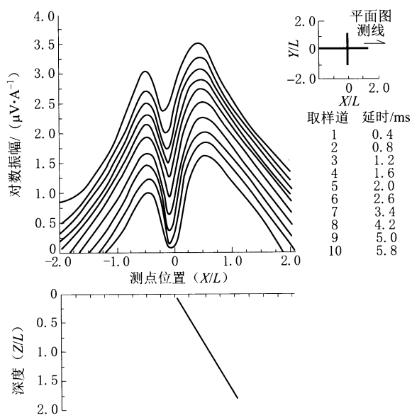
图 F.2 倾斜薄板模型的 TEM 曲线( \delta=60^\circ )
