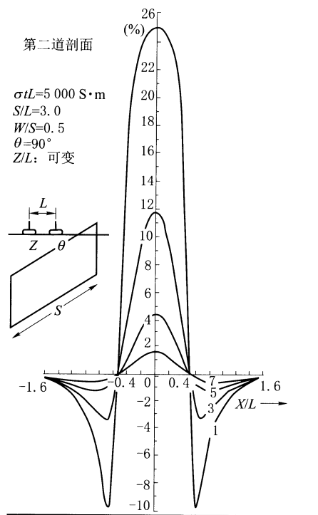
图 F.7 直立薄板埋深对 TEM 响应的影响
