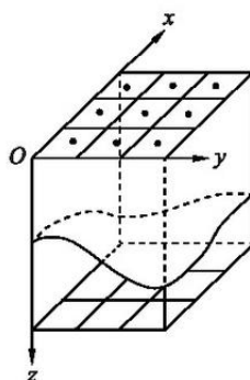
图 B.1 三维海底面直立六面体组合示意图
