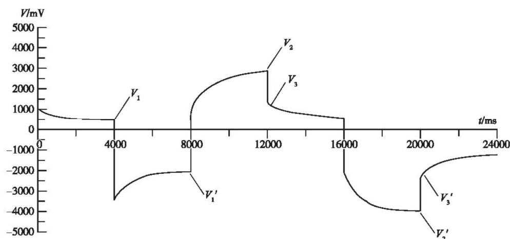
图1 样品架法测定岩矿石样品电性波形示意图
