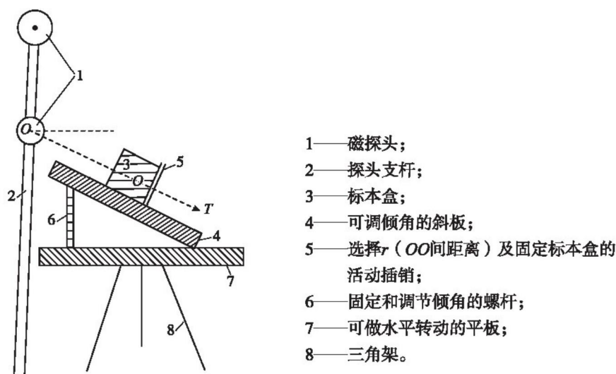
图 B.1 磁力仪测定岩矿石标本示意图
